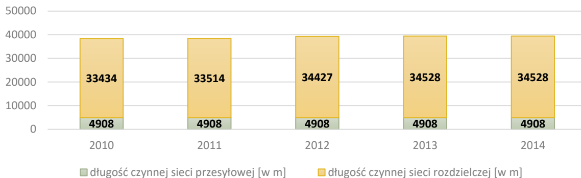
Wykres 17. Długość czynnej sieci gazowej w latach 2010-2014 na terenie gminy
