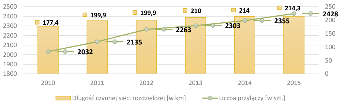
Wykres 13. Długość czynnej sieci wodociągowej i liczba przyłączy na terenie gminy w latach 2010-2015
